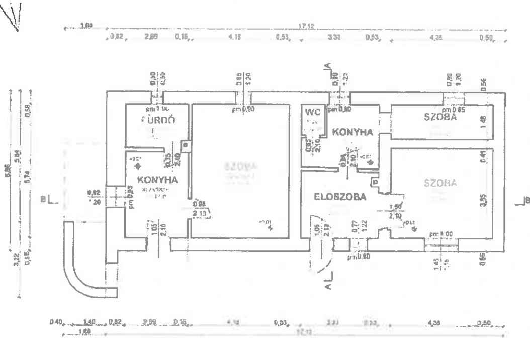
Az épület alaprajza
